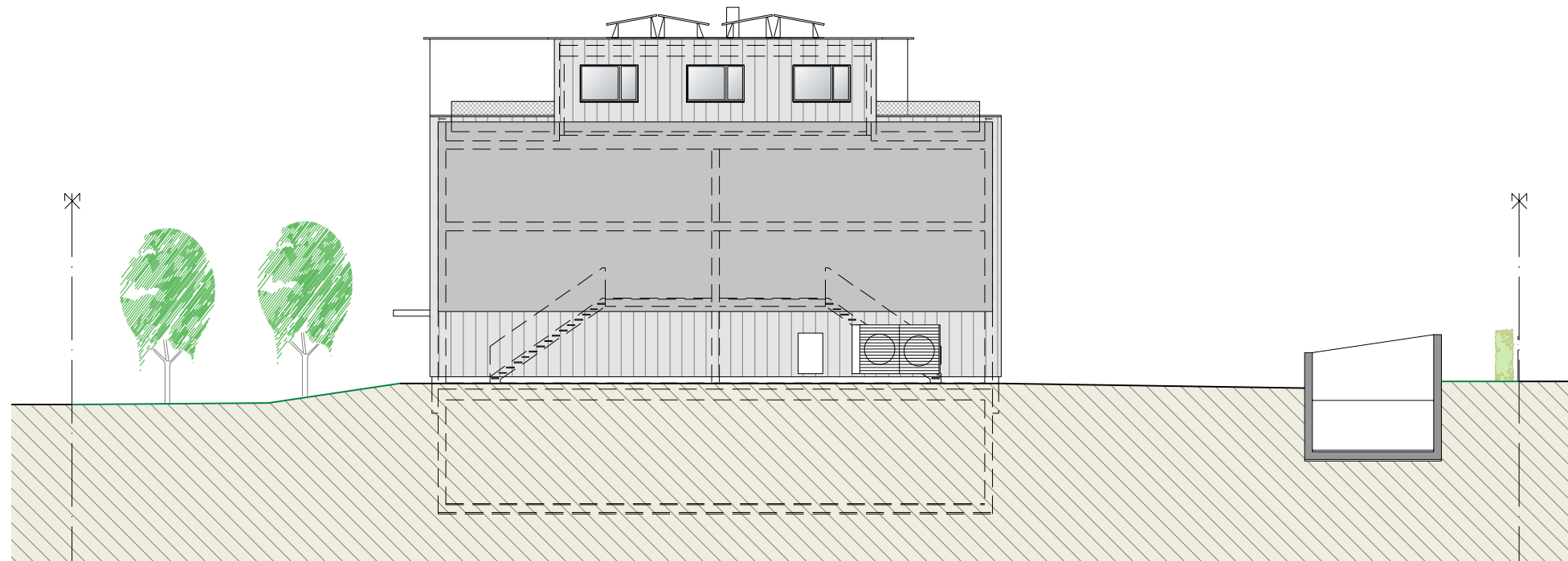
Südfassade
